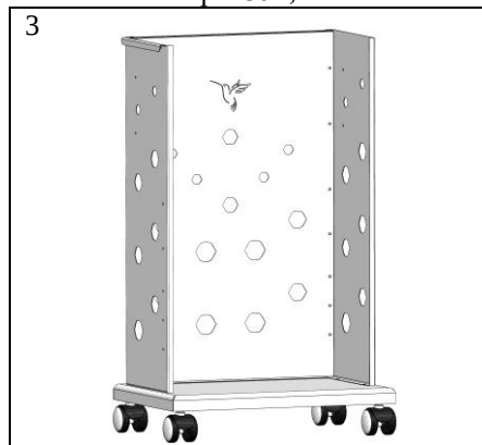
Велика панель всередині стійок, гвинт М4, шайба М4, гайка М4.
